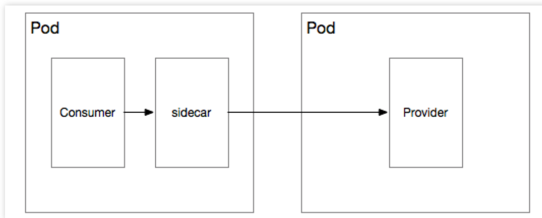
场景2：仅服务提供者作为 Mesh 应用部署
