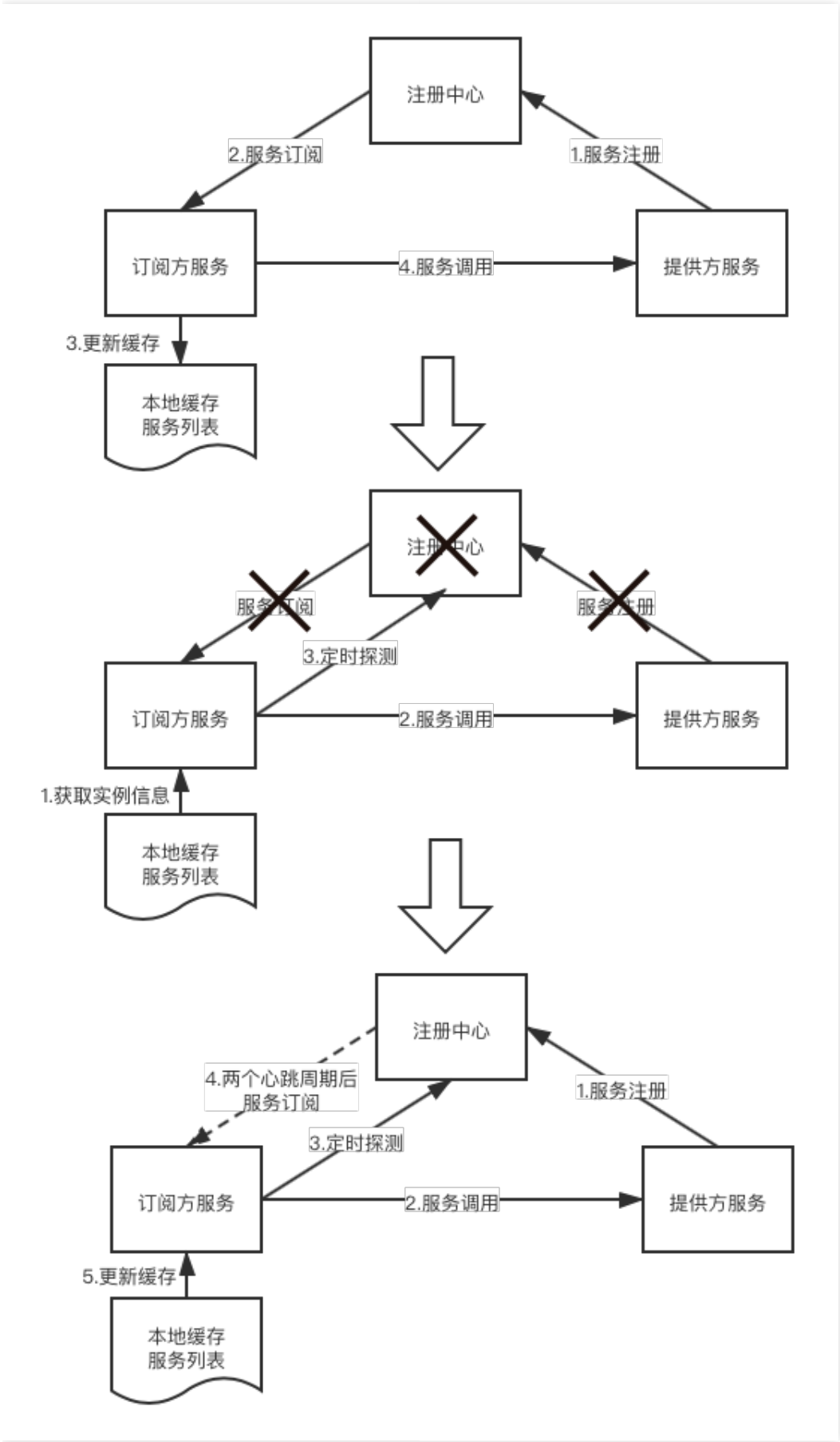
正常状态服务调用流程：
