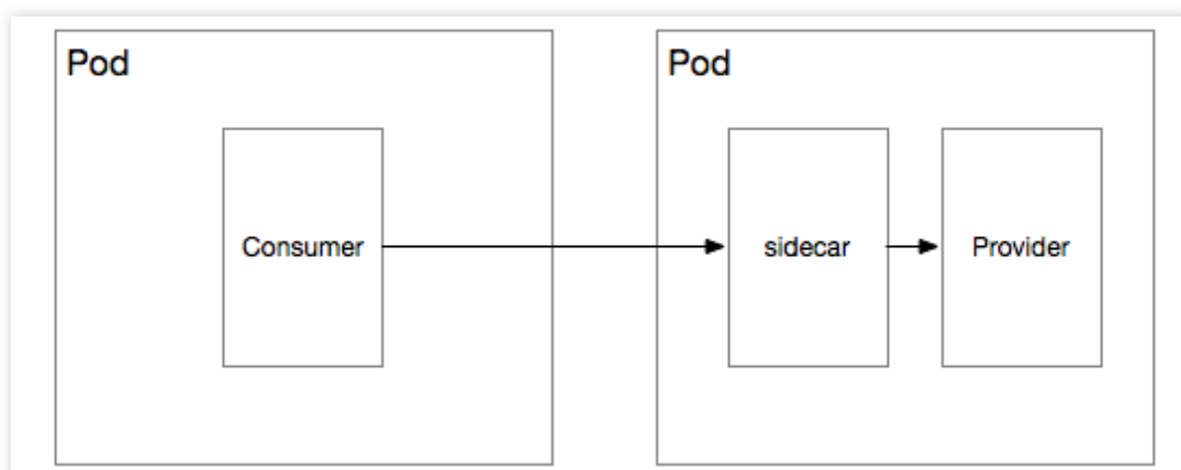
场景3：服务消费者和服务提供者均作为 Mesh 应用部署
