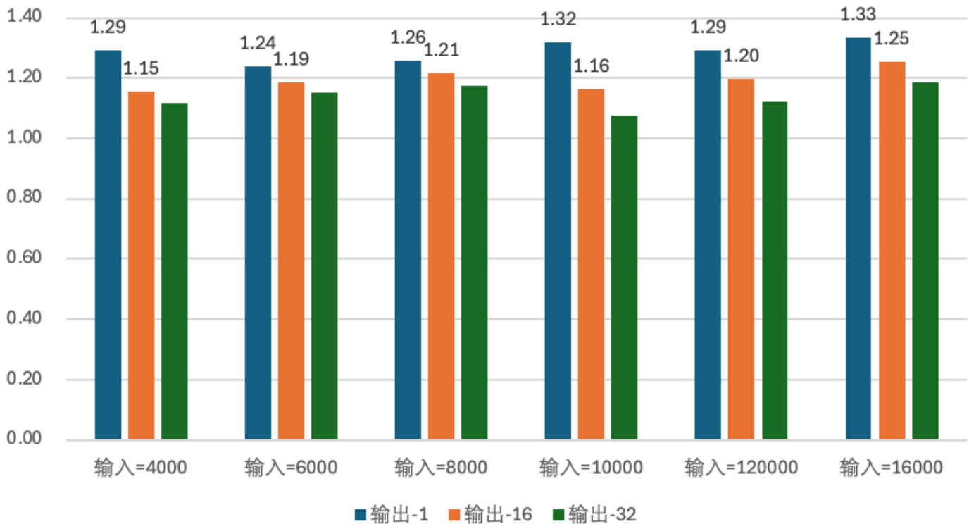
L20不同输入输出SP相对于TP收益 (FP8)
