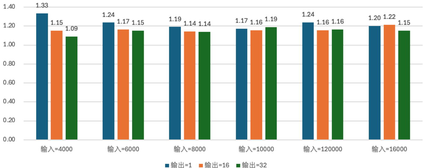
FP8 SP相对于TP性能 (Llama3-8B)
